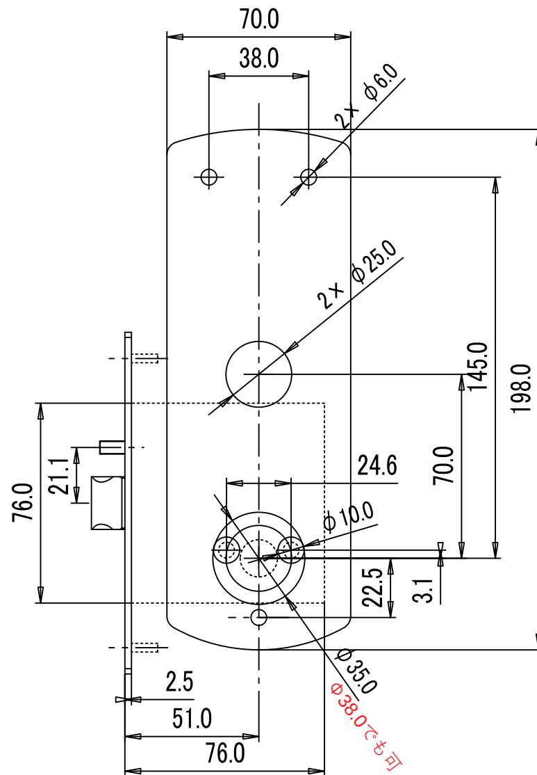
Escutcheon & Lockcase
